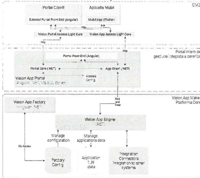
Figură 1 – Arhitectura aplicație
