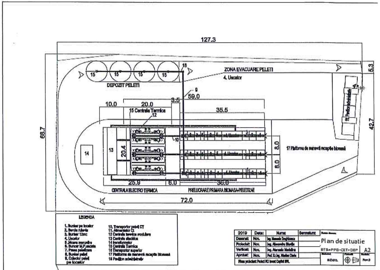
A2 Plan de situatie BTB-CET
