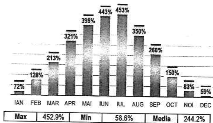
Acoperire solară (%)
