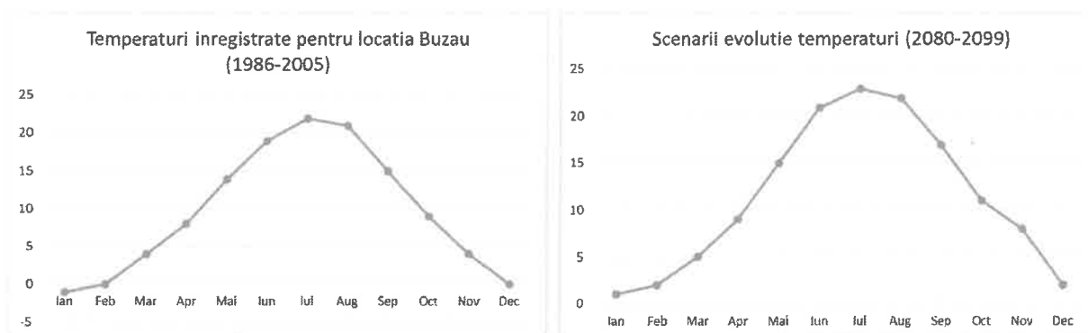
Fig. 2.14. Compararea temperaturilor înregistrate în perioada 1986 - 2005 cu scenariile de temperaturi corespunzătoare perioadei 2080 - 2099
