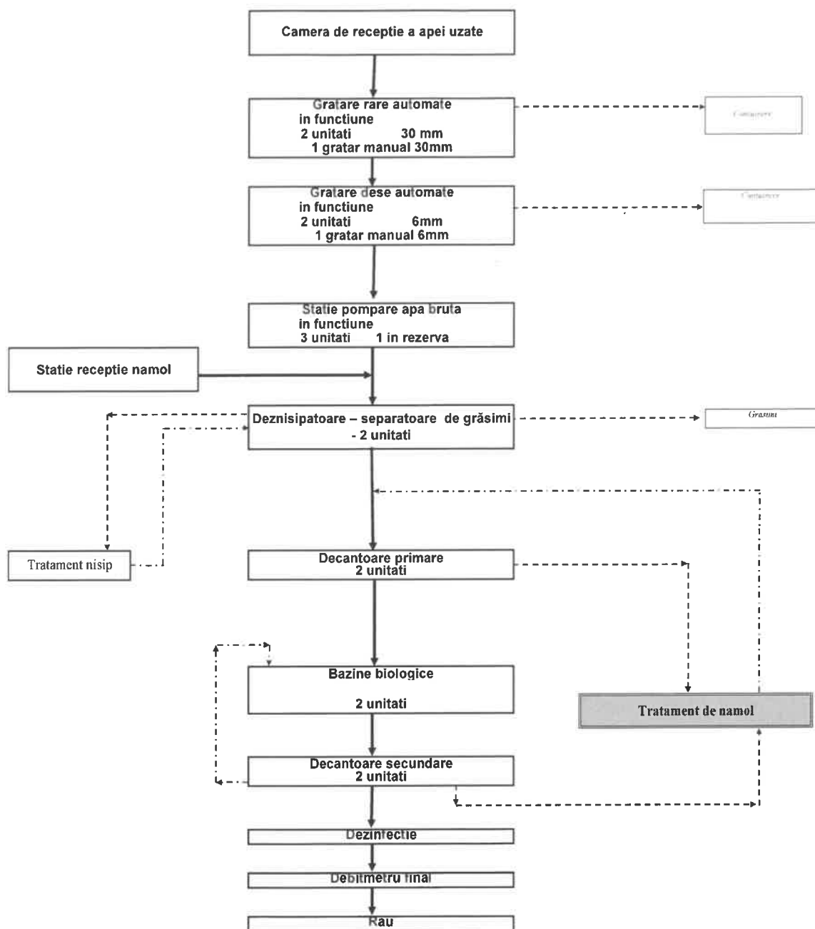
Schema 2.1. Diagrama fluxului tehnologic-Filiera de tratare a apei
