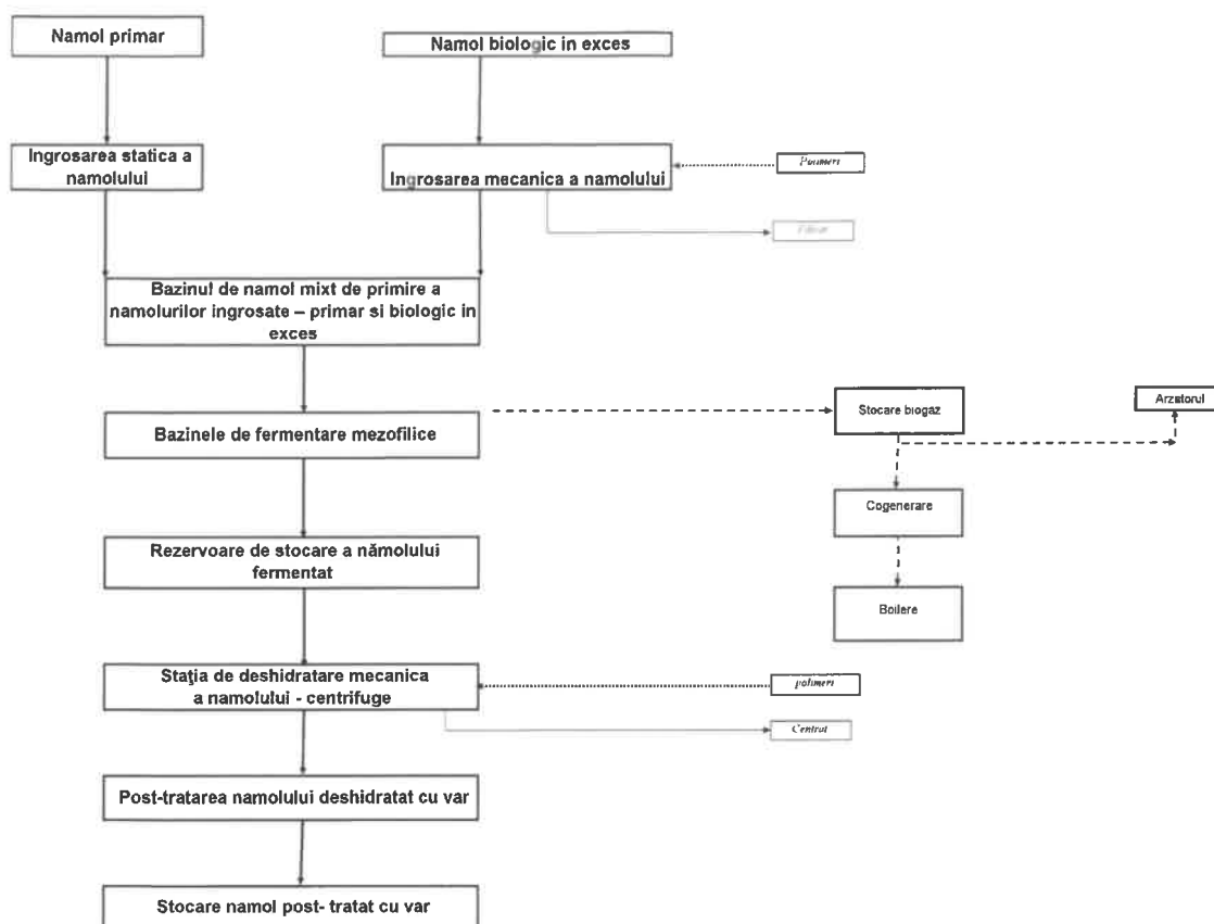
Schema 2.2. Diagrama fluxului tehnologic-Filiera de tratare a nămolului
