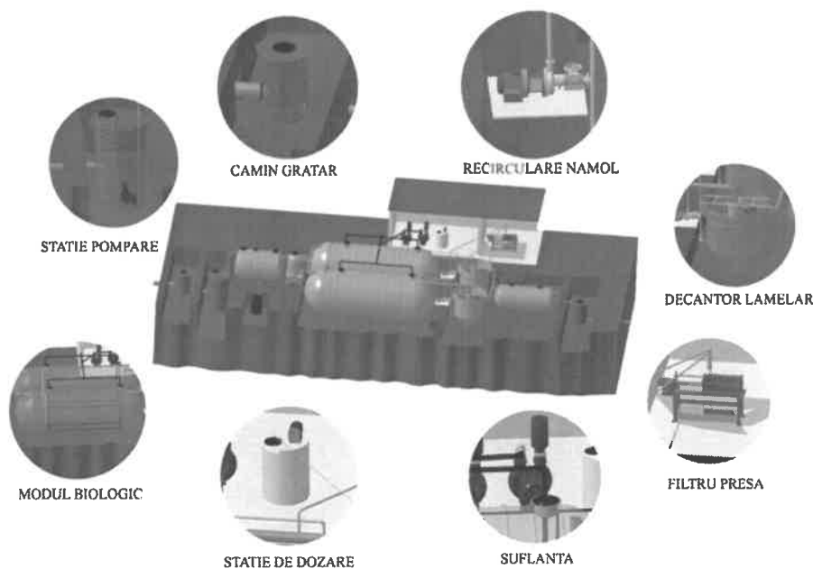
Fig. 2.7. Stație de epurare municipală – model
