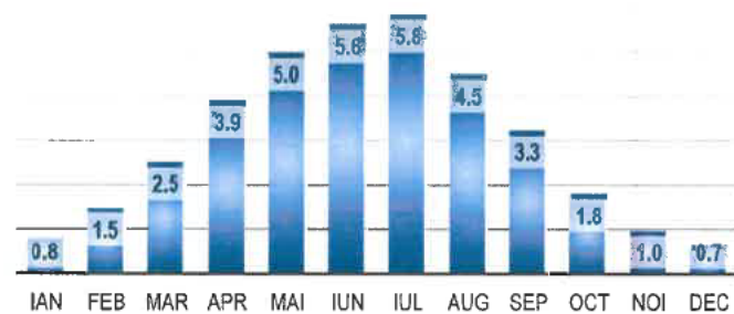
Radiatia solara pe plan inclinat (kWh/zi)
